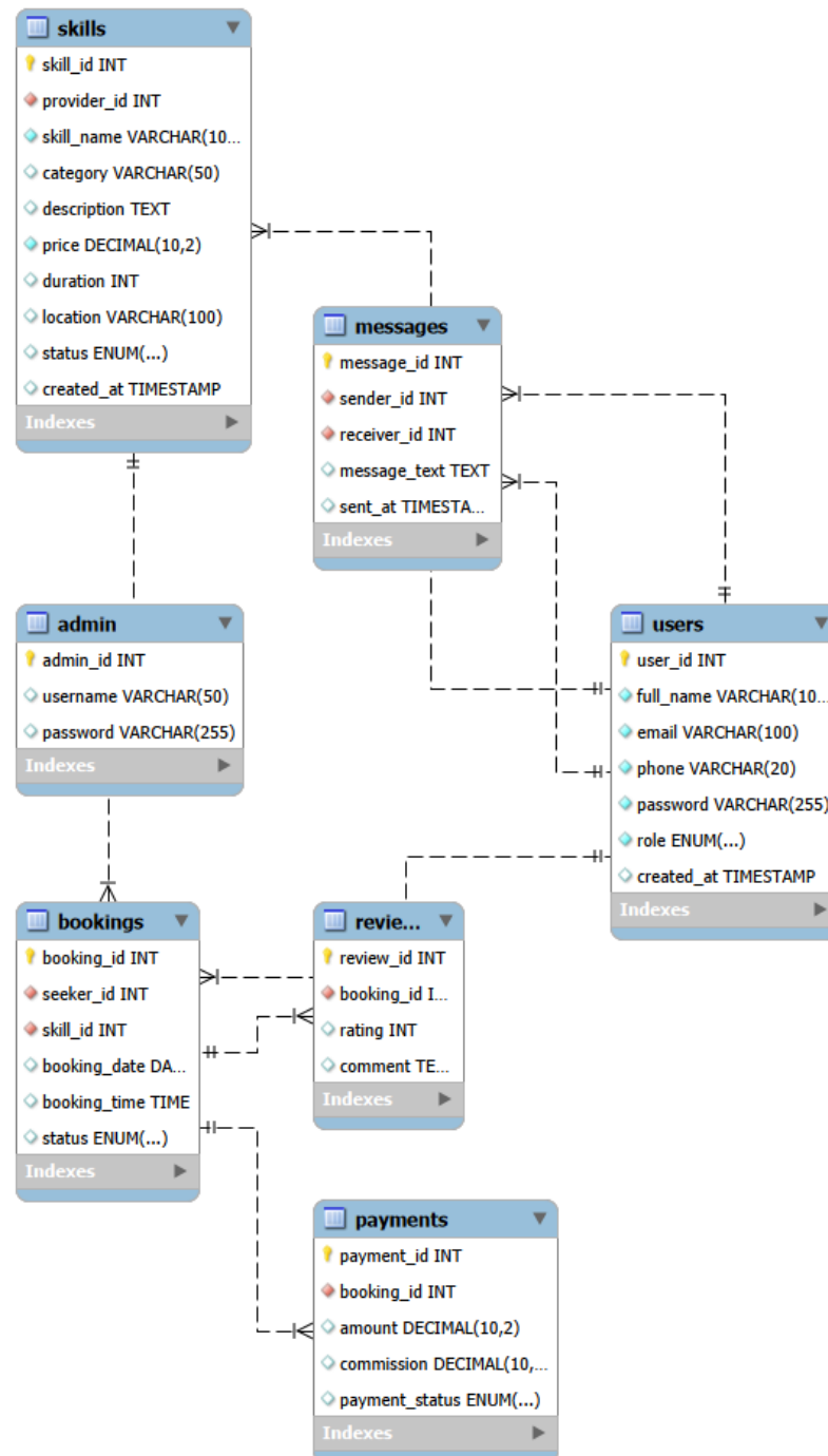
Figure 4: ER Diagram
